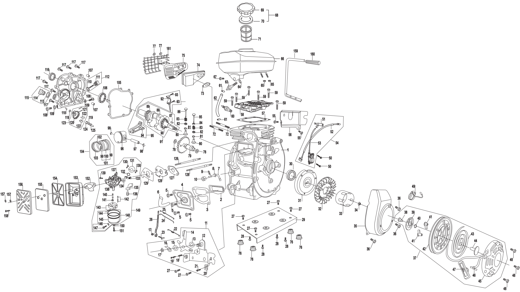
152F-3爆炸图
